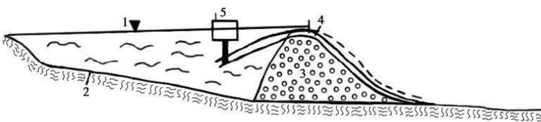
ნახ. 1. ხეობის ჩახერგილი წყალდაგუბების უბანი და მისი საფონური წყალამოღვის სქემა.
