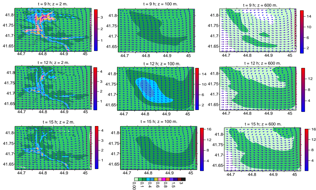
ნახ. 2. ფდ სუსტი ქარის დროს ქარის სიჩქარისა (მ/წმ) და მტერის კონცენტრაციის (ზდკ) განაწილება, როცა t = 9, 12 და 15 სთ მიწის ზედაპირიდან 2, 100 და 600 მ სიმაღლეებზე
