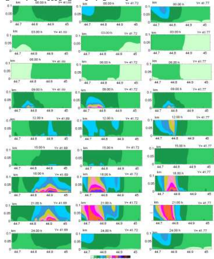
ნახ. 8. ფდ სუსტი ქარის დროს ერთი დღე-ღამის განმავლობაში მტვრის კონცენტრაციების (ზდკ) განაწილება ატმოსფეროს მიწისპირა ფენაში პარალელის გასწვრივ მდებარე სამ ვერტიკალურ სიბრტყეში ( Y= 41.69°, Y=41.72° და Y=41.77°)
