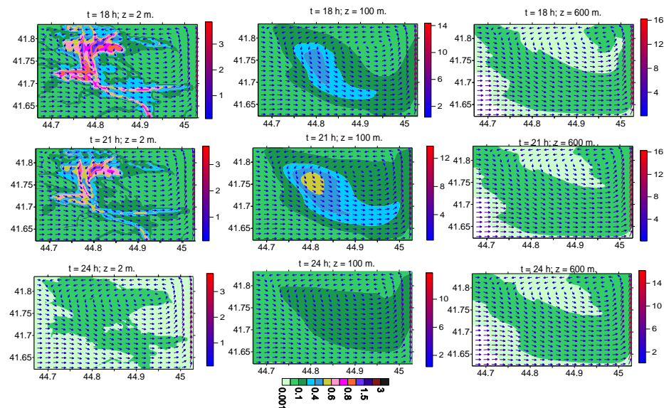
ნახ. 3. ფდ სუსტი ქარის დროს ქარის სიჩქარისა (მ/წმ) და მტერის კონცენტრაციის (ზდკ) განაწილება, როცა t = 18, 21 და 24 სთ მიწის ზედაპირიდან 2, 100 და 600 მ სიმაღლეებზე
