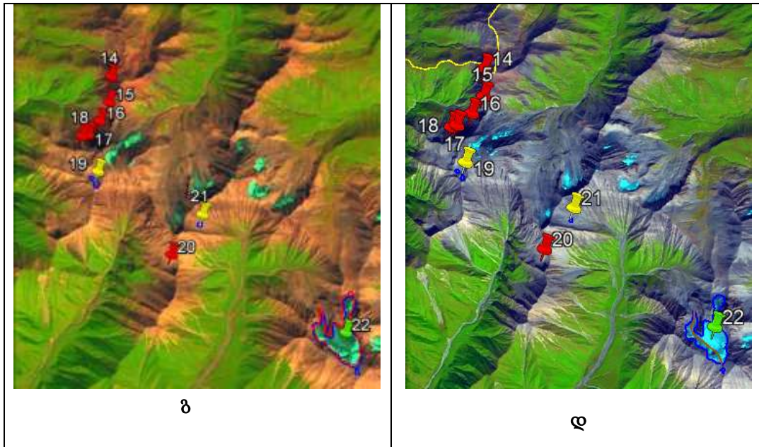
სურ. 2. მდ. ლიახვის აუზის მცინვარების დეგრადაციის ამსახველი სურათები. ქემელთასა და მომაგდონის ხეობაში მდებარე №1-13 მცინვარების და სბადონისა და კალასანიდონის ხეობაში მდებარე №14-22 მცინვარების ვიზუალიზაცია და კონტურები. ინფორმაცია განსაზღვრული LANDSAT 8-ის 2014 წლის 28 აგვისტოს (თდზ 1 (ა და გ)) და 2020 წლის 13 სექტემბერის (თდზ 2 (ბ და დ)) თანამგზავრული სურათების საფუძველზე
