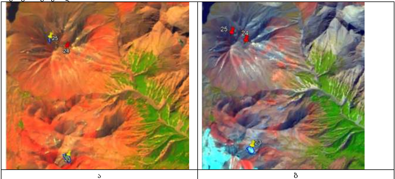
სურ. 3. მდ. მტკვრის მარცხენა შენაკადის, თეთრი არაგვის აუზში მდებარე მცირე მდინარეები №23-26 მცირე მდინარეების ვიზუალიზაცია და კონტურები განსაზღვრული Landsat-ის თანამგზავრული სურათის მიხედვით: ა – თდზ 1; ბ – თდზ 2
