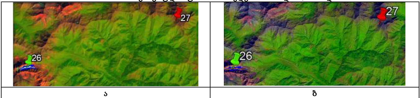
სურ. 4. მდ. მტკვრის მარცხენა შენაკადის, ხევსურეთის არაგვის მარჯვენა შენაკადის აბუდელაურის ხეობაში მდებარე №26 აბუდელაურის და №27 მცირე მდინარეების ვიზუალიზაცია და კონტურები განსაზღვრული Landsat-ის თანამგზავრული სურათის მიხედვით: ა – თდზ 1; ბ – თდზ 2
