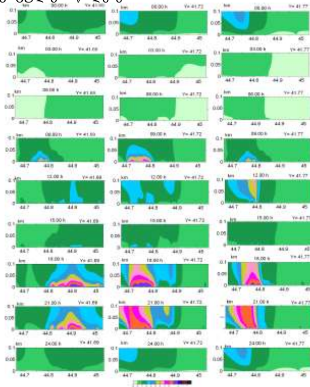
ნახ. 8. ფდ სუსტი ქარის დროს ერთი დღე-ღამის განმავლობაში მტვრის კონცენტრაციების (ზდგ) განაწილება ატმოსფეროს მიწისპირა ფენაში პარალელის გასწვრივ მდებარე სამ ვერტიკალურ სიბრტყეში ( Y = 41.69^{\circ} , Y = 41.72^{\circ} და Y = 41.77^{\circ} )
