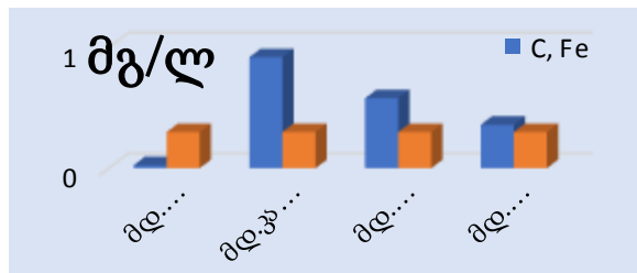
გრაფიკი 3. Fe-ის საშუალო წლიური შემცველობები მდინარეებში - ფოლადაური, კაზრეთულა, მაშავერა, ხრამი
