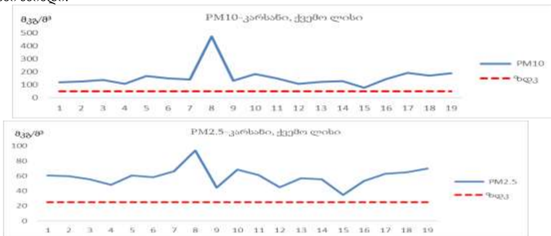
ნახ. 11. PM 2.5 და PM 10 კონცენტრაციები კარსანი-ქვემო ლისის გზის მონაკვეთზე
