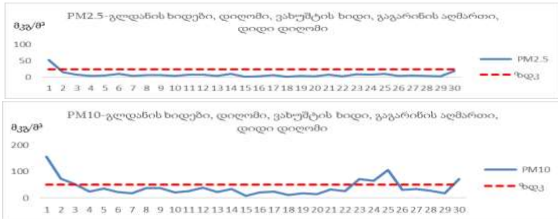
ნახ. 10. PM 2.5 და PM 10 კონცენტრაციები გლდანის ხიდები-დიდი დილომის გზის მონაკვეთზე
