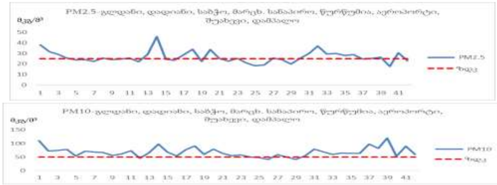
ნახ. 9. PM 2.5 და PM 10 კონცენტრაციები გლდანი-დამბალოს გზის მონაკვეთზე
