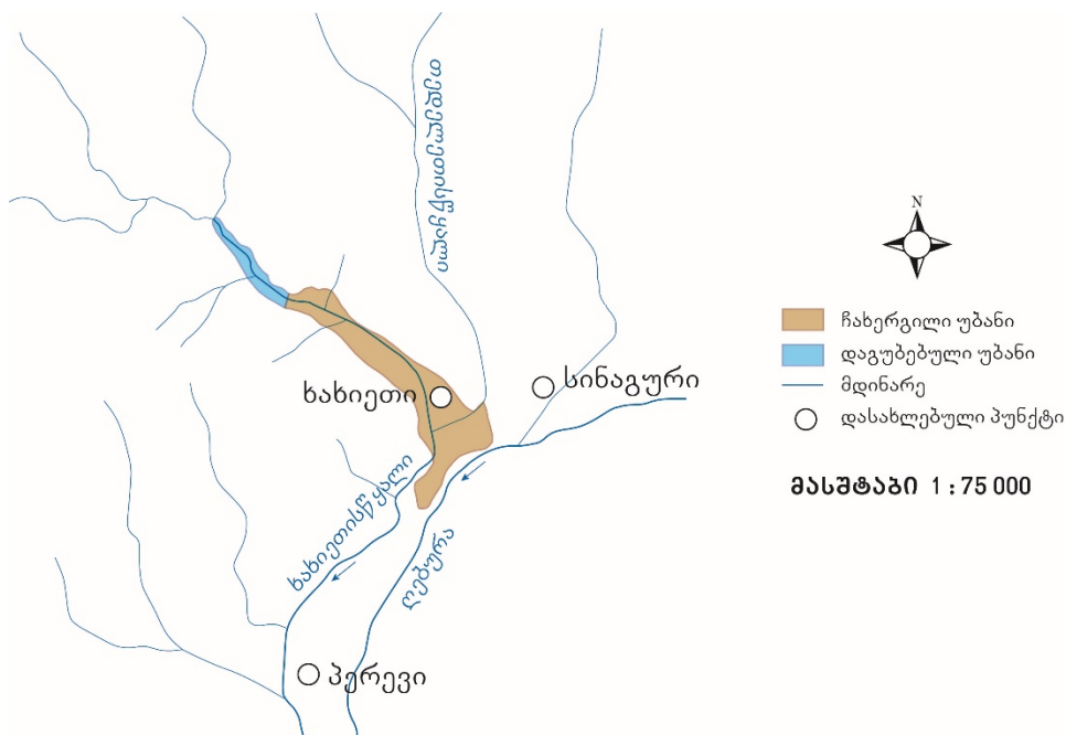
ნახ. 25. მდ. სახიეთისწყლის კლდე-ზვავით ჩახერგილი უბანი (ვ. ცომაია, 1991 წ.)
