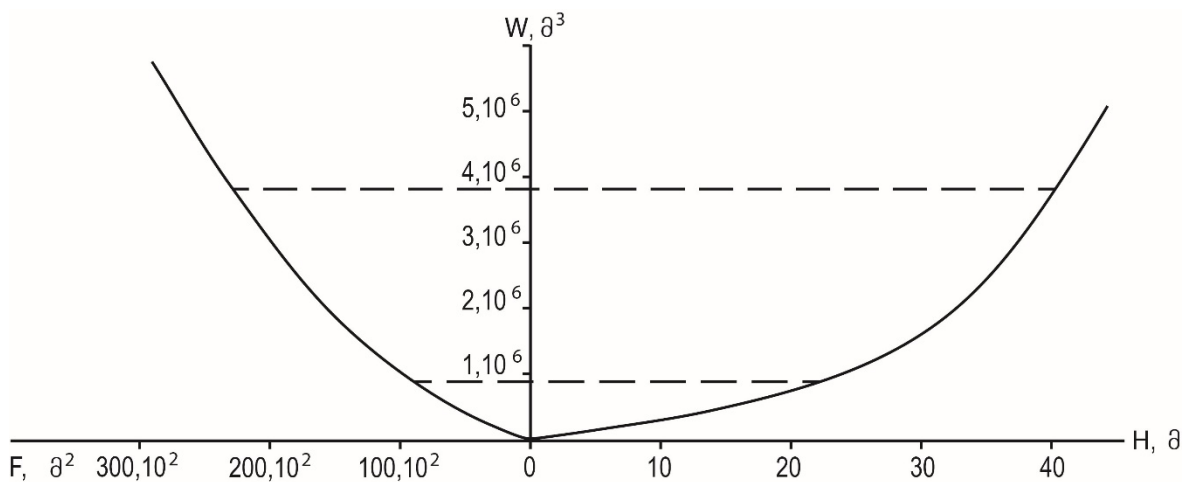
ნახ. 31. მდ. ფაწას დაგუბებული ტბის მოცულობის (W), სარკის ფართობის (F) და მეწყრული კაშხლის სიმაღლის (H) ურთიერთდამოკიდებულების გრაფიკები.
